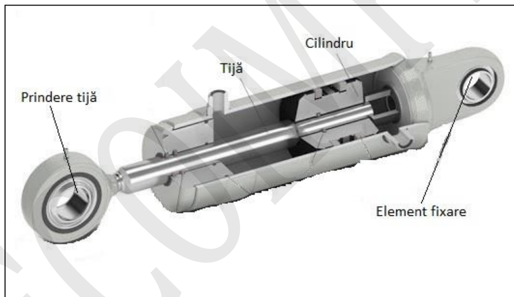
Fig. 1. Cilindru hidraulic
